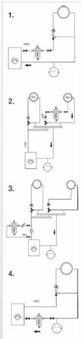
Montagebeispiel: vertikale Leitung
